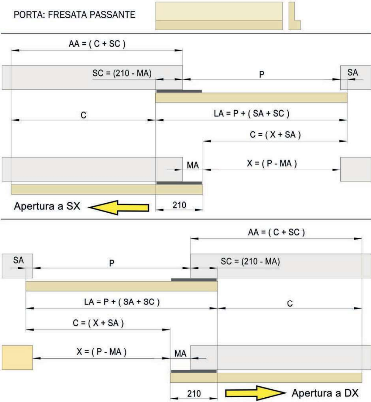
AIRONE FRESATA PASSANTE: Tabella calcolo
