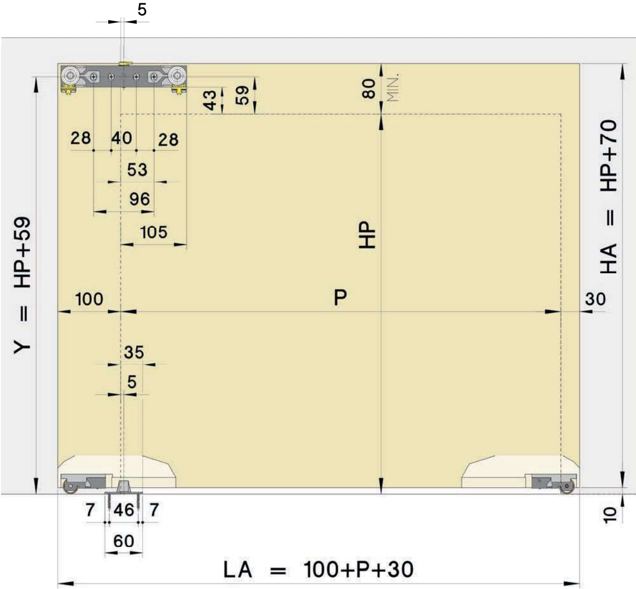
Apertura Parziale Porta a SX, per Maniglione
