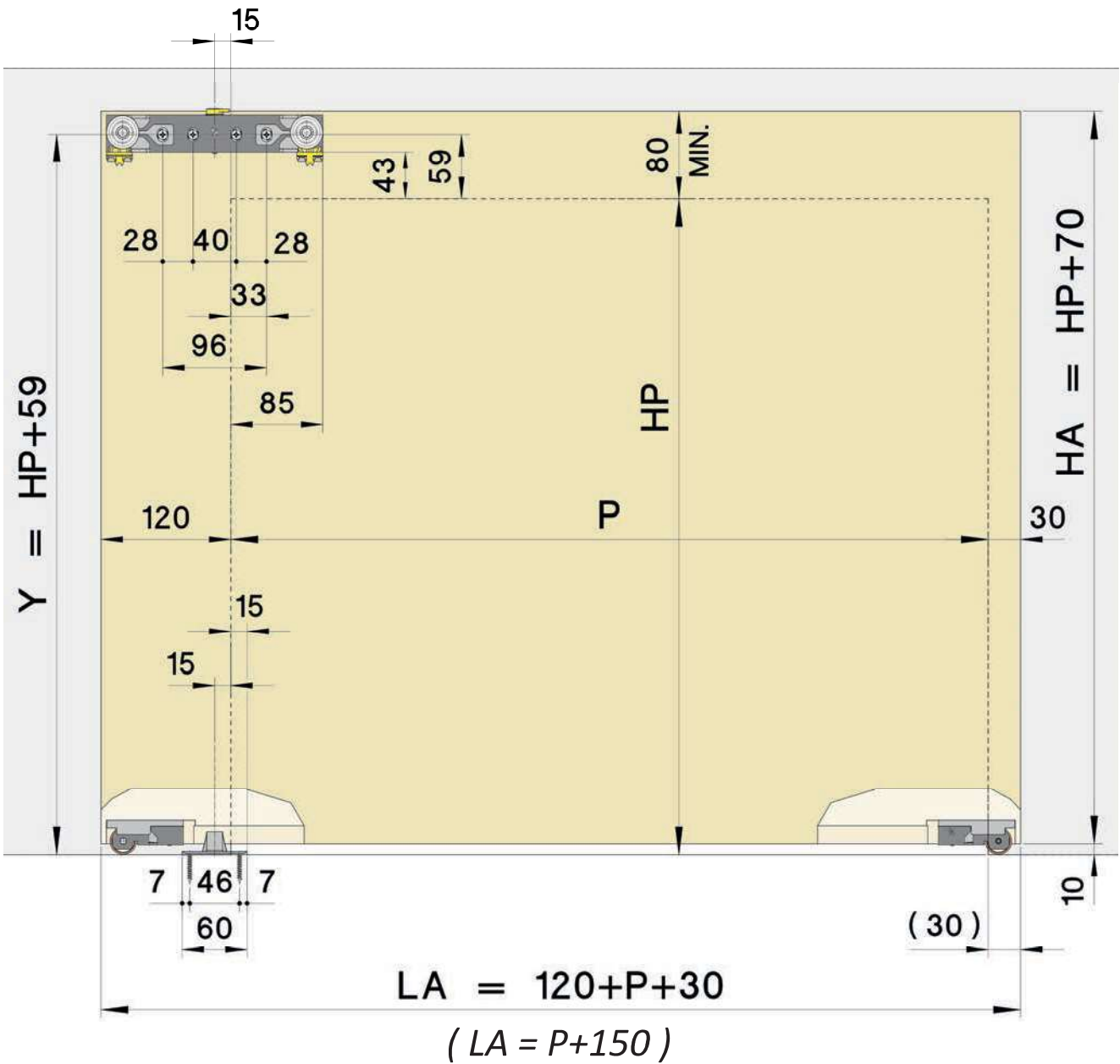
Apertura Parziale Porta a SX, posizione STANDARD
