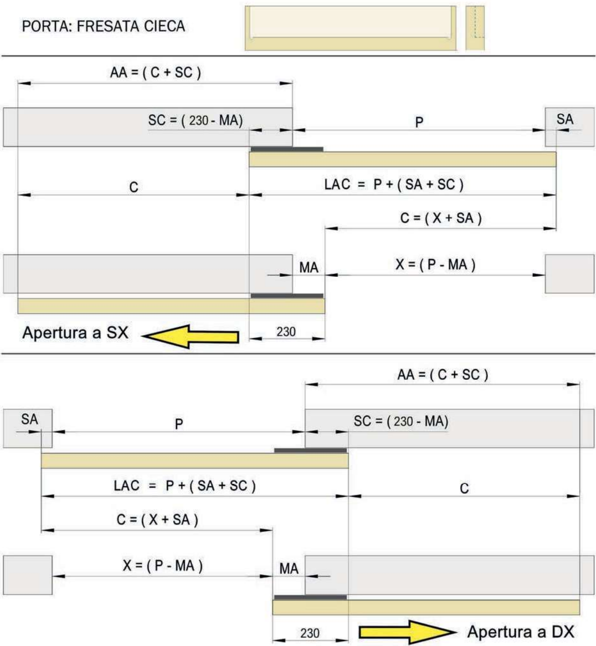
AIRONE FRESATA CIECA (non passante): Tabella calcolo
