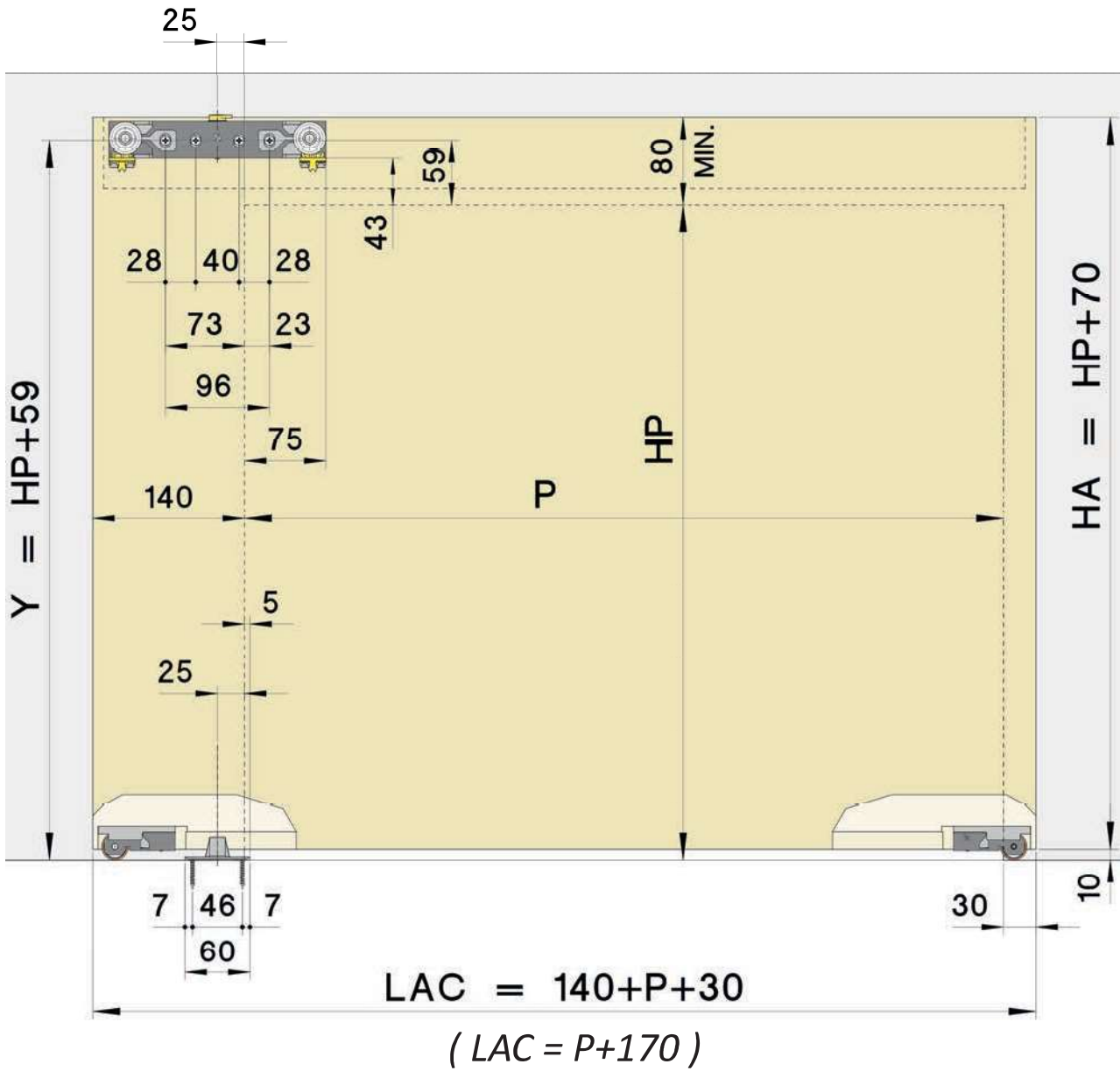
Apertura Parziale Porta a SX, posizione STANDARD
